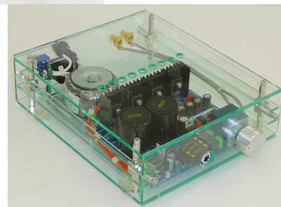
アクリルケースに組み込んだ製作例
