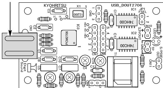
CN1 USBコネクタ
