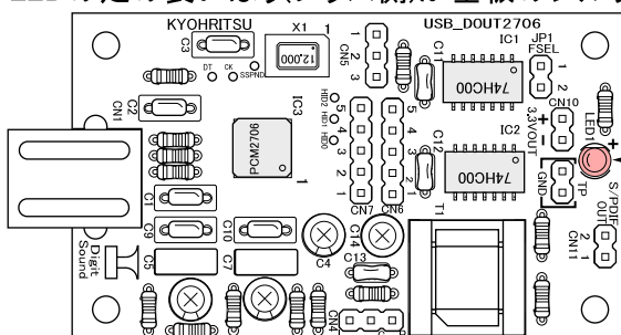
LED1 LED(3φ、赤)
