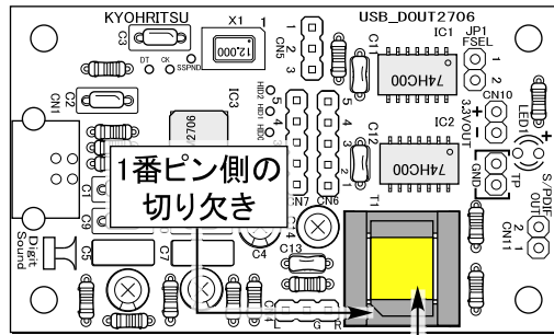
T1 パルストランス
