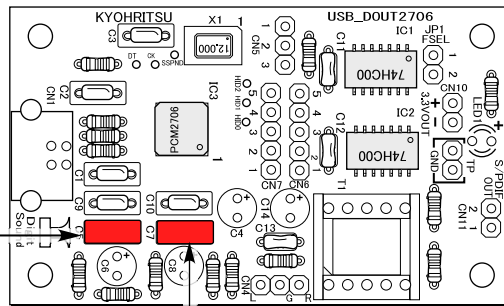
C5 フィルムコンデンサ 0.022 \mu F C7 フィルムコンデンサ 0.022 \mu F(223)
