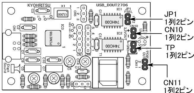
基板上的ヘッダピンのシルク印刷
