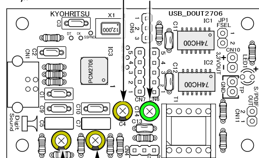
C4 電解コンデンサ 50V 10 \mu F C14 バイポーラ電解コンデンサ (BP) 16V 10 \mu F
