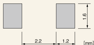
マウントパッド
