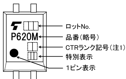
図 14.1 TLP620M 現品表示例
