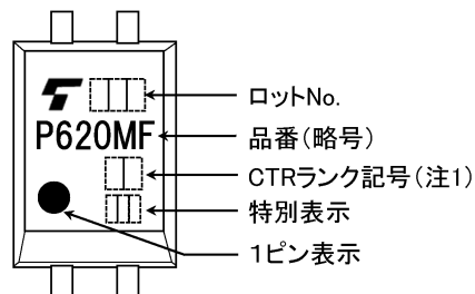
図 14.2 TLP620MF 現品表示例
