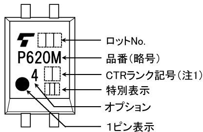
図 15.4 TLP620M 現品表示例 (注)
