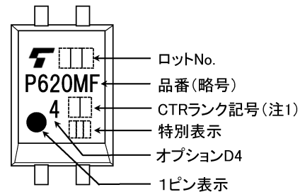
図 15.5 TLP620MF 現品表示例 (注)
