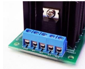
←左からGND、M-、M+、E+、VCC
