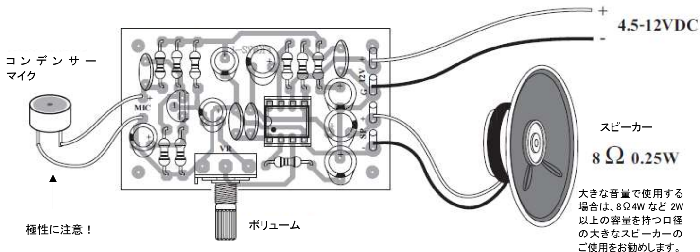
実体配線図
