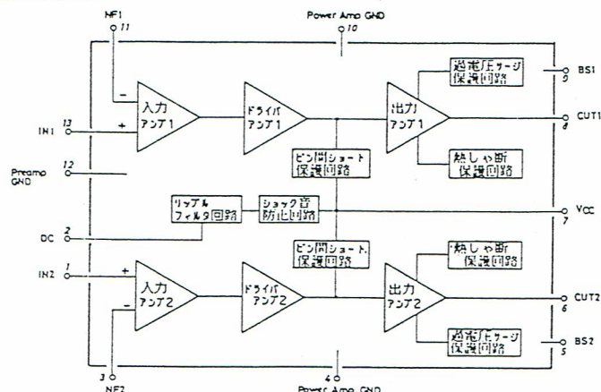
等価回路ブロック図
