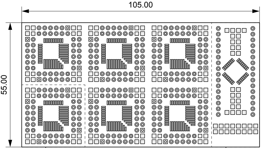
基板外形図
