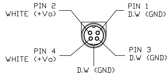
4P POWER DIN FRONT VIEW
