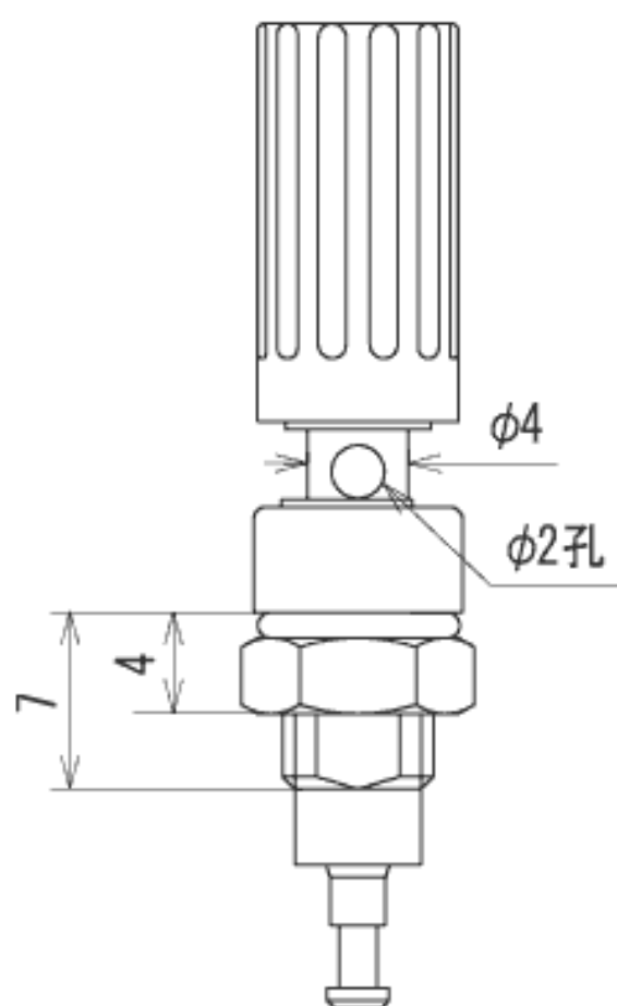
取付孔寸法例
