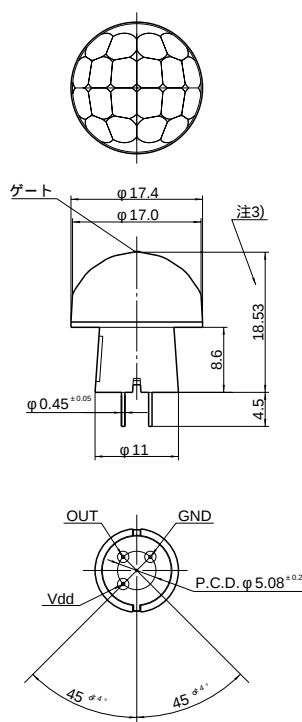
外形寸法図
