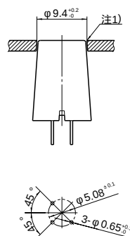
推奨穴加工寸法
