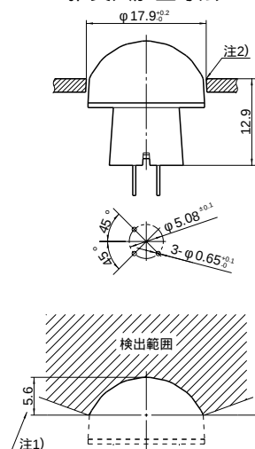
推奨穴加工寸法
