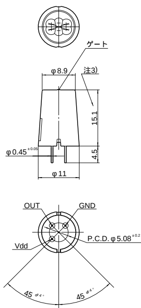
外形寸法図
