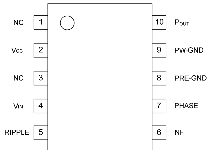
SSOP-10
