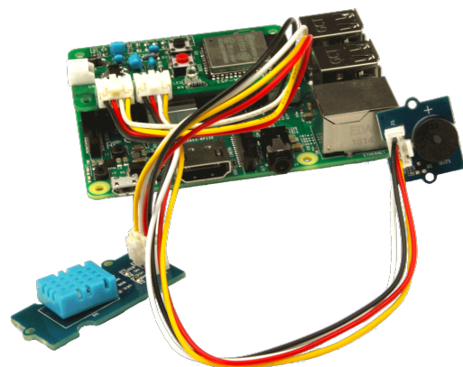
接続例：温湿度センサー+ブザー
