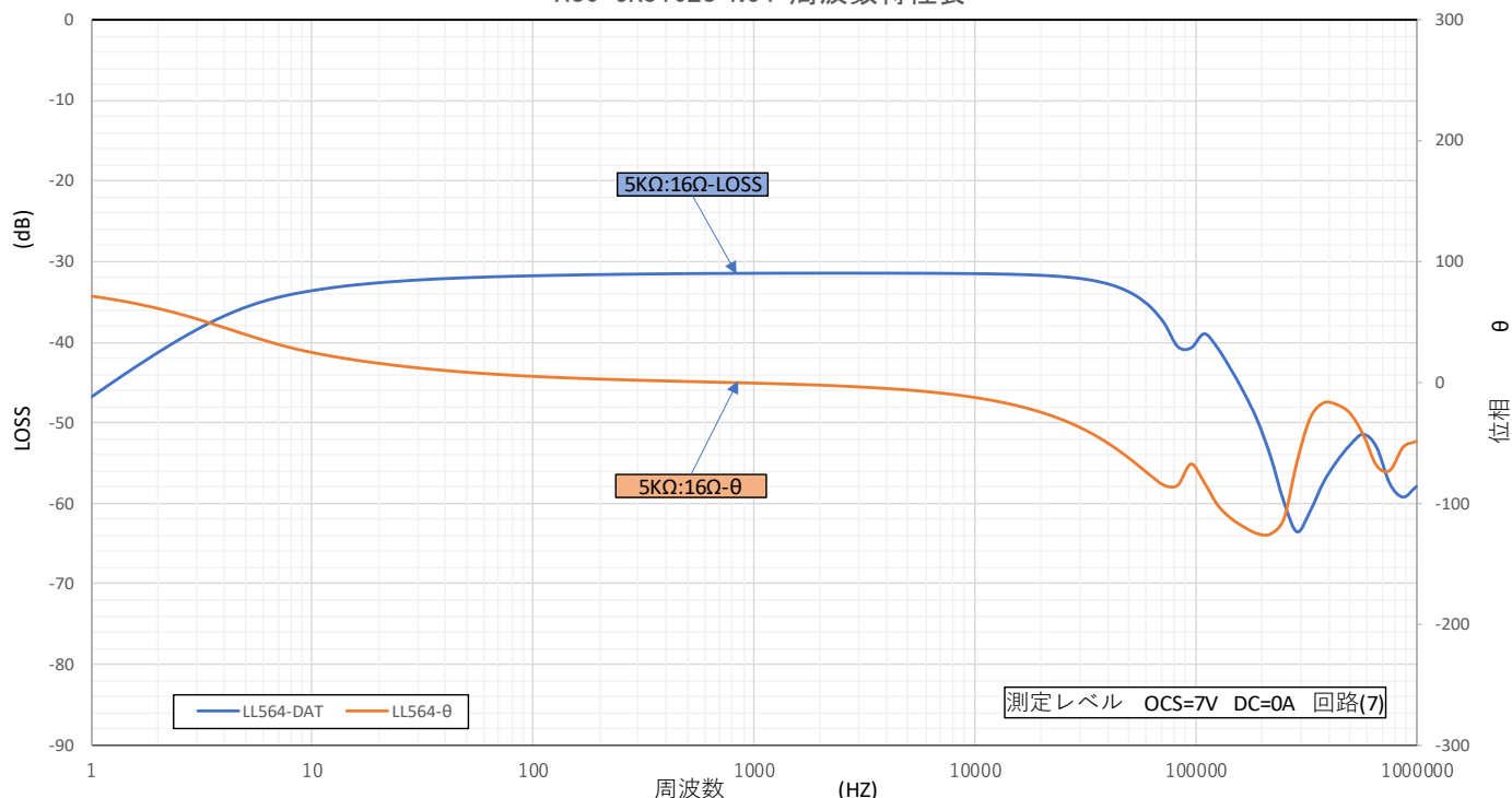
A86-5K816LS N04 周波数特性表
