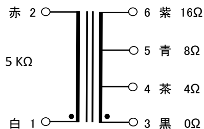
接続図
